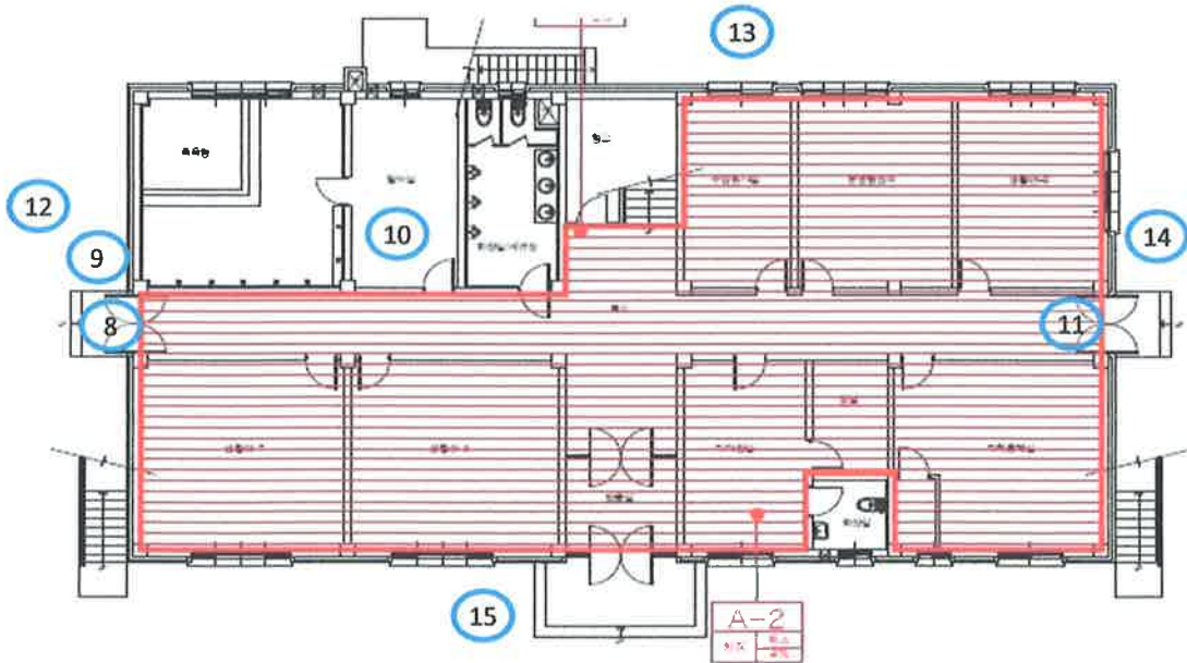
명영생활관 1층 평면도
