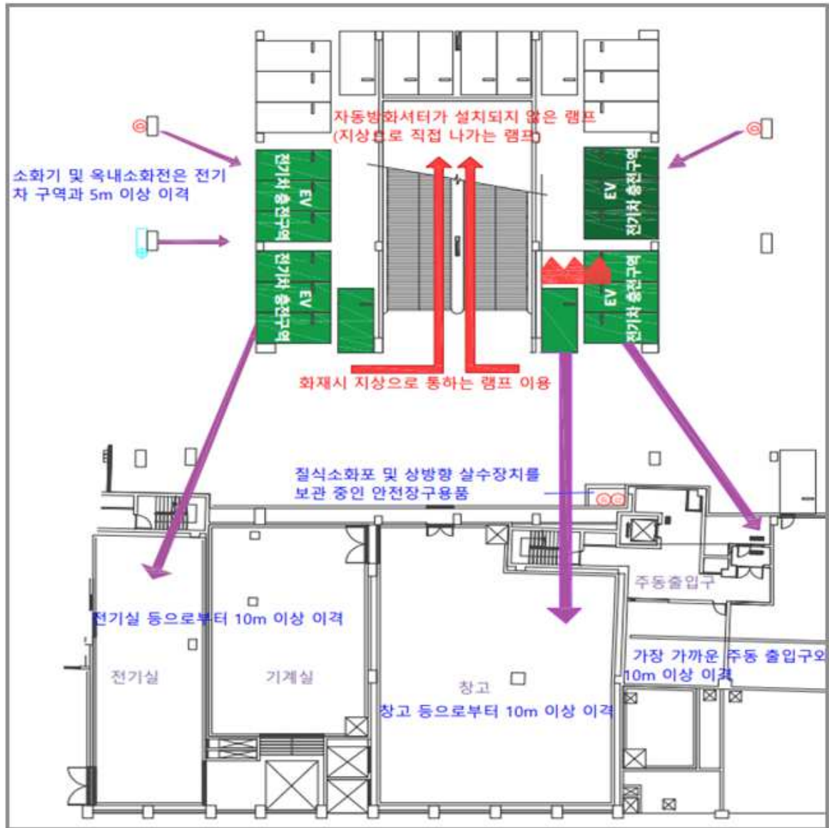
<그림 11> 전기차 충전구역 소방·안전시설 지하주차장 배치도 예시
